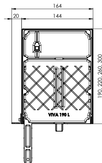
Řez příznaného boxu VIVA + P 020/02, P 080/02, P 081/02
