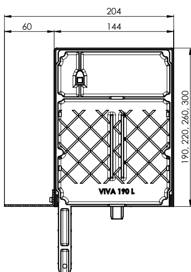
Řez přiznaného boxu VIVA + P 020/06, P 080/06, P 081/06 190 x 140b 220 x 140b 260 x 140b 300 x 140b
