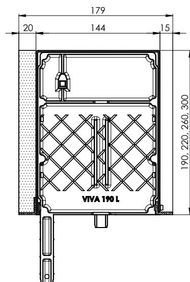
Řez zaomítacího boxu VIVA
