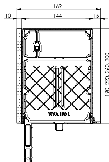
Řez zaomítacího boxu VIVA 190 x 169 x 2L x STY10 220 x 169 x 2L x STY10 260 x 169 x 2L x STY10 300 x 169 x 2L x STY10
