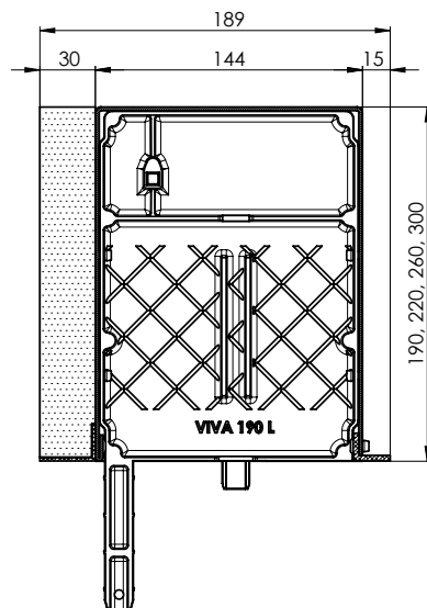
Řez zaomítacího boxu VIVA
