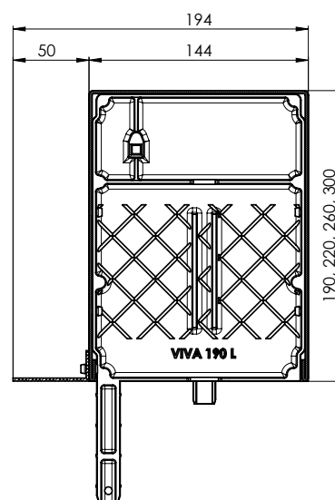
Řez příznaného boxu VIVA + P 020/05, P 080/05, P 081/05
