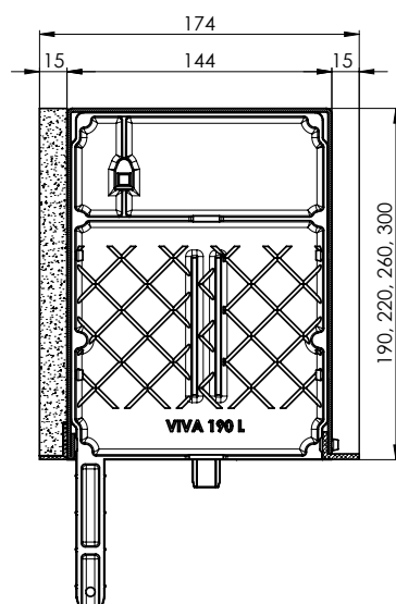
Řez zaomítacího boxu VIVA
