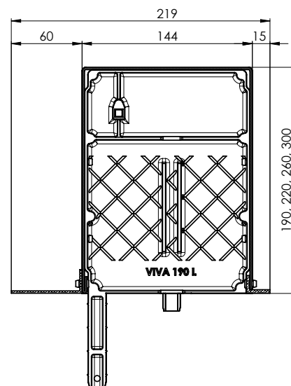
Řez zaomítacího boxu VIVA + P 020/06, P 080/06, P 081/06 190 x 150Lb 220 x 150Lb 260 x 150Lb 300 x 150Lb
