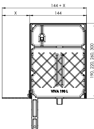
Řez přiznaného boxu VIVA + P 020/07-20, P 080/07-20, P 081/07-20 190 x 140b 220 x 140b 260 x 140b 300 x 140b
